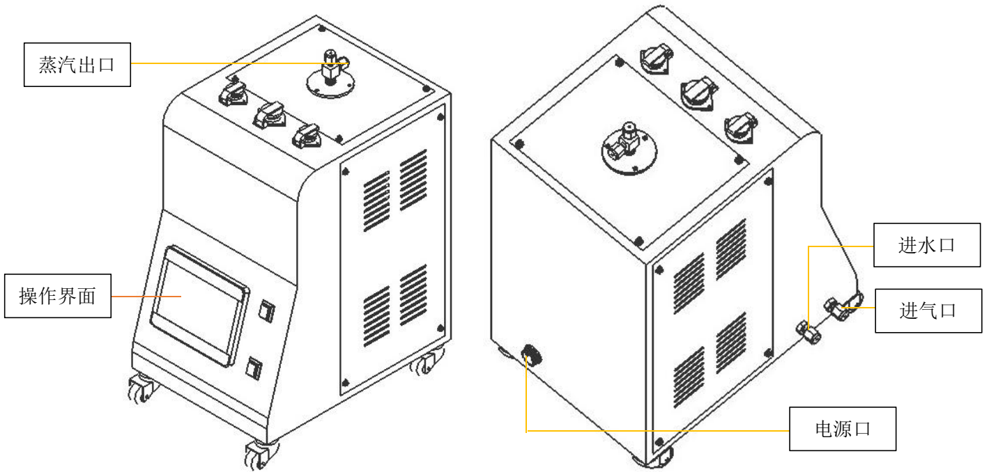
HSG01 空间布置图
