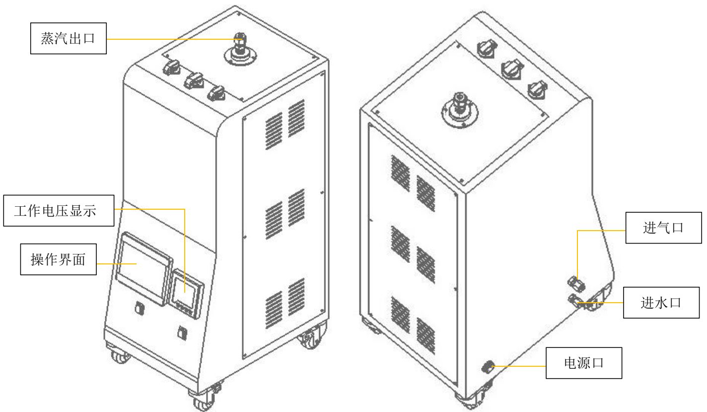
HSG10 空间布置图
